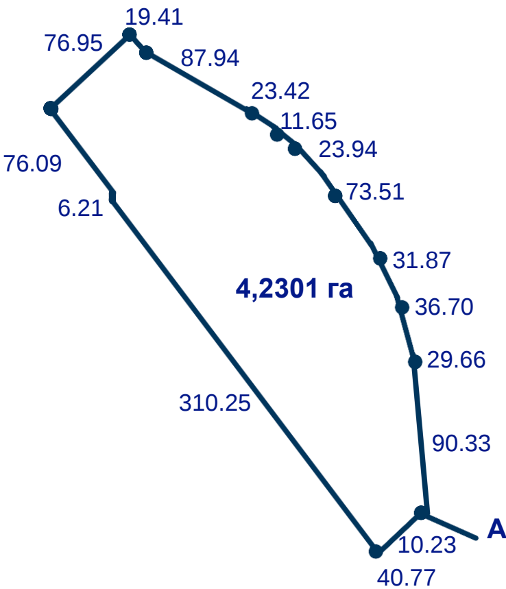
План меж земельної ділянки к/н 7110400000:03:001:0006
