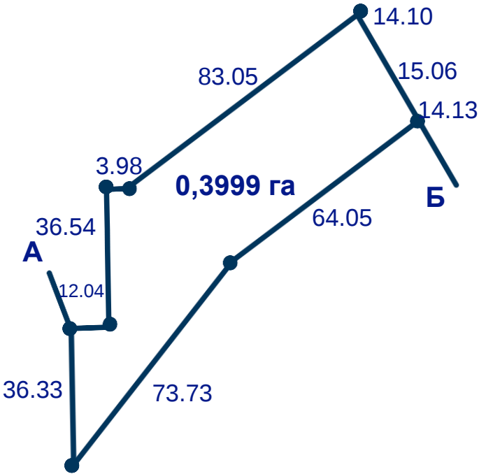
План меж земельної ділянки к/н 7110400000:03:001:0008
